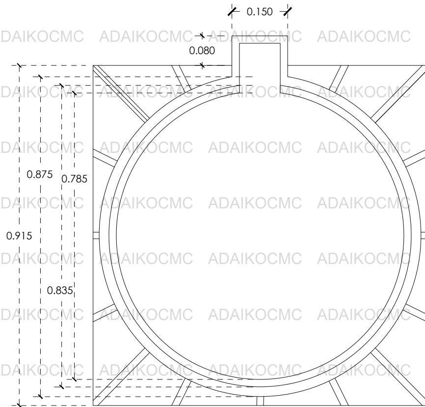
ARO SIN TAPA EN PLANTA
