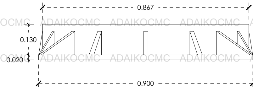
PERFIL DE ARO
