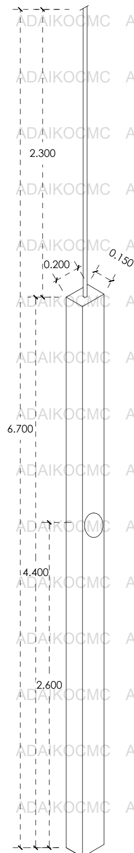
ISOMÉTRICO POSTERIOR
