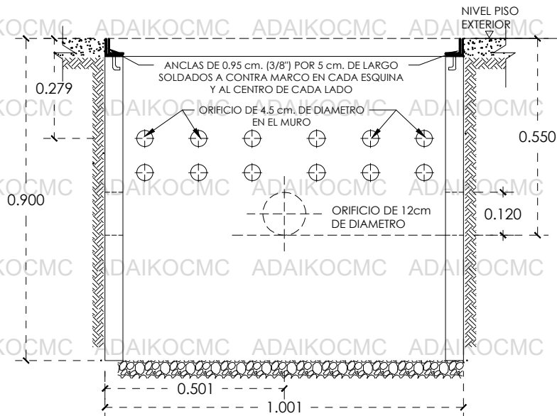
REGISTRO SIN FONDO PARA NIVEL FREATICO BAJO, CORTE A-A'
