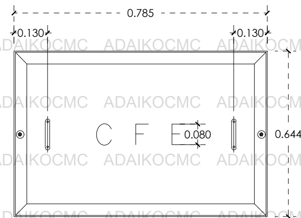
PLANTA TAPA
