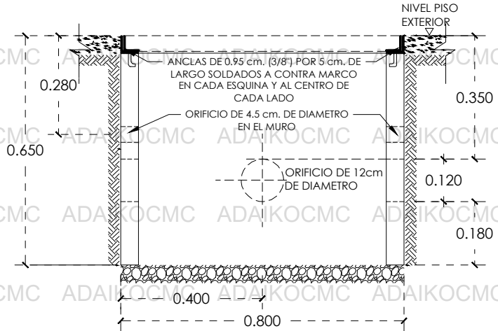
REGISTRO SIN FONDO PARA NIVEL FREATICO BAJO, CORTE A-A'
