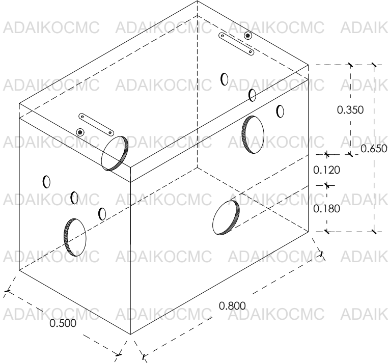
ISOMETRICO
