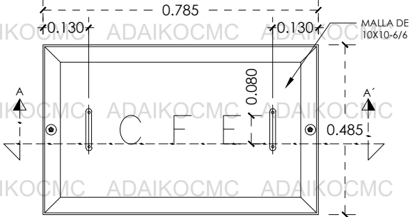
PLANTA TAPA
