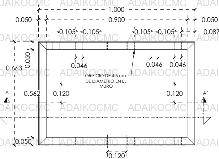
PLANTA REGISTROSIN FONDO
