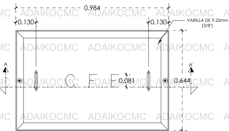
PLANTA TAPA
