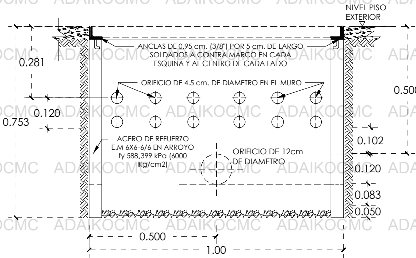
REGISTRO SIN FONDO PARA NIVEL FREATICO BAJO, CORTE A-A'
