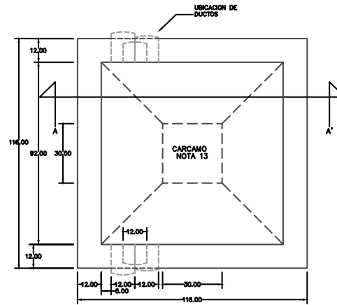
PLANTA PISO
