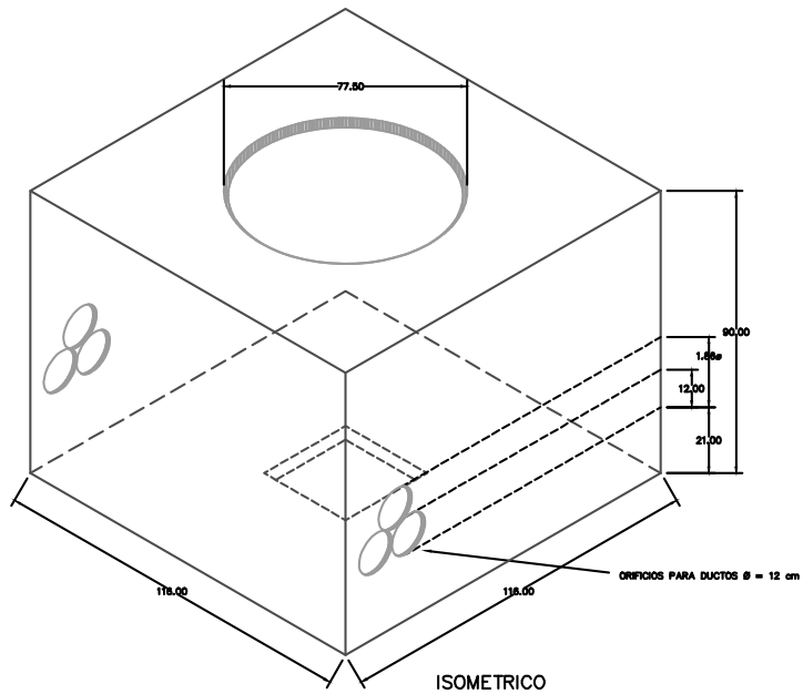
ISOMETRICO
