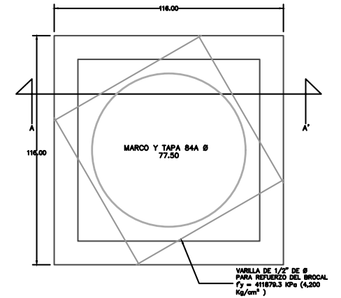
PLANTA TAPA
