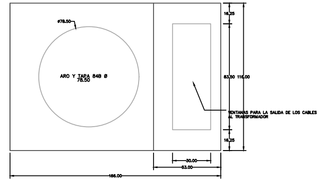
PLANTA TAPA
