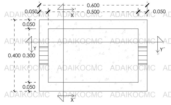
PLANTA DE REGISTRO SIN FONDOS Y TAPA
