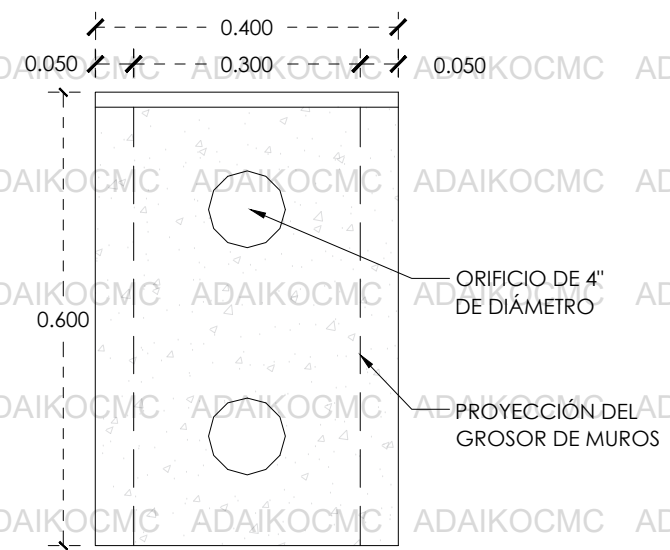
CORTE TRANSVERSAL X-X' REGISTRO SIN FONDO PARA NIVEL FREÁTICO BAJO
