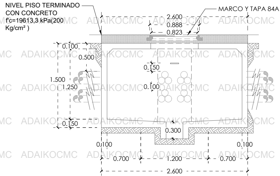
ELEVACION REFUERZO SECCION A-A' ESC. 1:40
