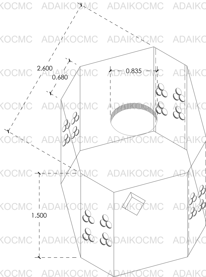
ISOMETRICO ESC. 1:40
