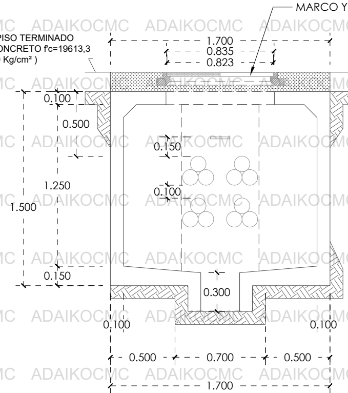
ELEVACION REFUERZO SECCION A-A'
