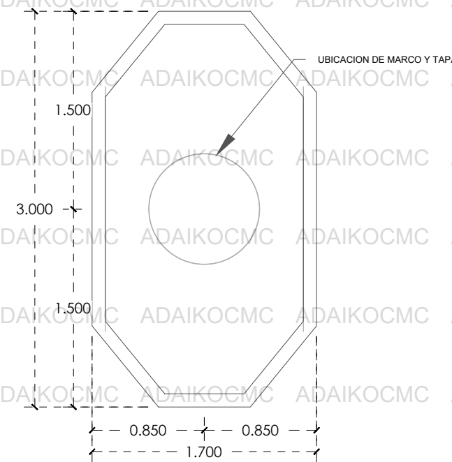
REFUERZO EN LOSA SUPERIOR
