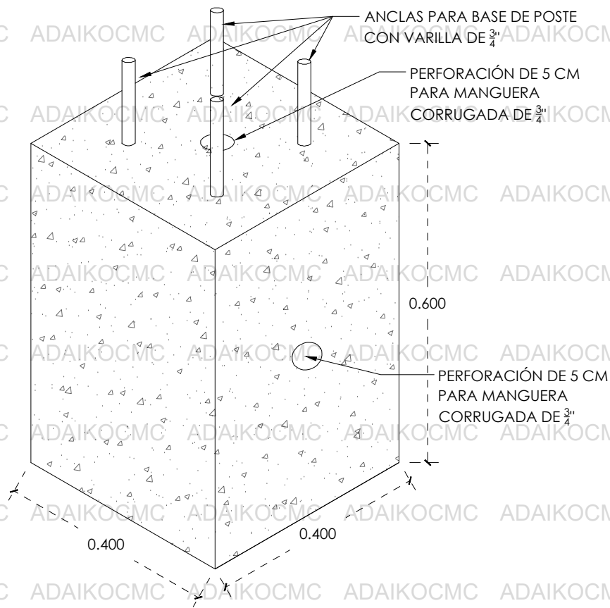
ISOMÉTRICO
