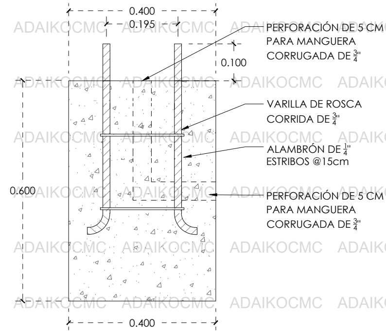
CORTE
