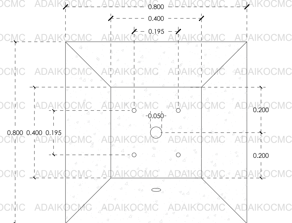
PLANTA
