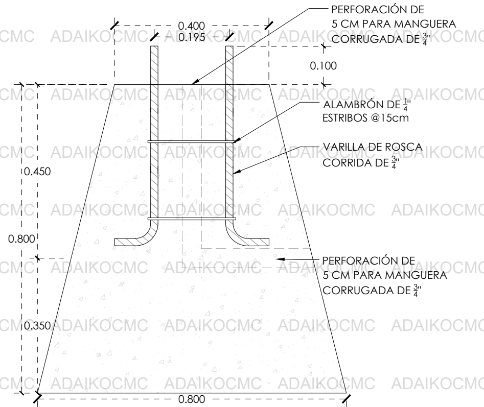
CORTE
