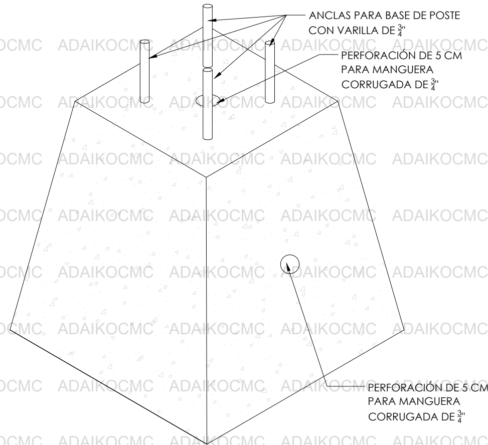
ISOMÉTRICO
