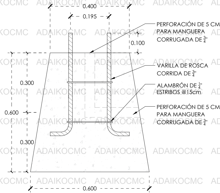
CORTE
