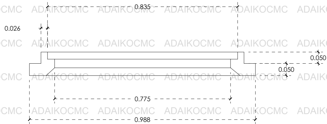
TUERCA GALVANIZADA DIAM. 12.7 mm, AHOGADA EN EL CÓLADO
